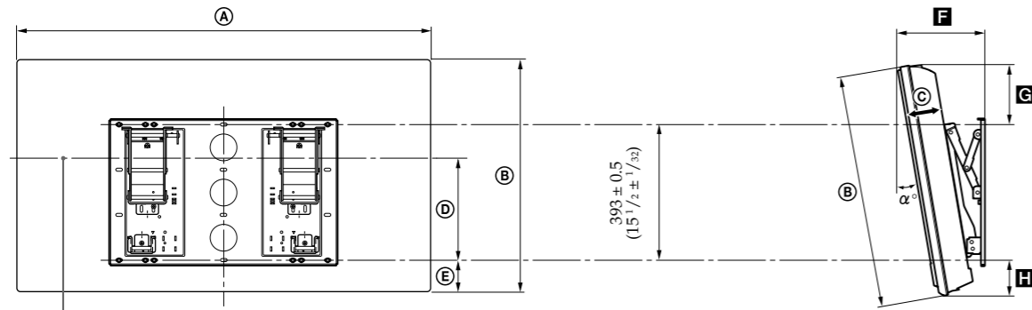
Center line of the screen when installed on the wall/ Axe central de l'écran lorsqu'il est installé au mur
