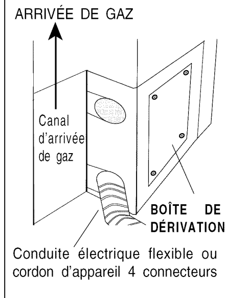
FIG. 9 – Emplacement de la boîte de dérivation sur les cuisinières mixtes.
