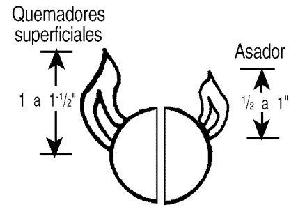
FIG. 17 – Llama correcta (Aprox.)
