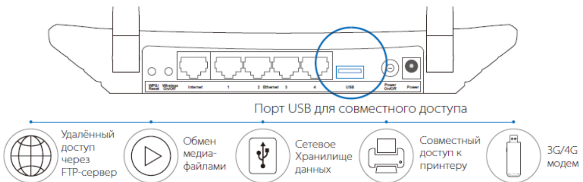
Рис. 2-1 Подключение устройств
