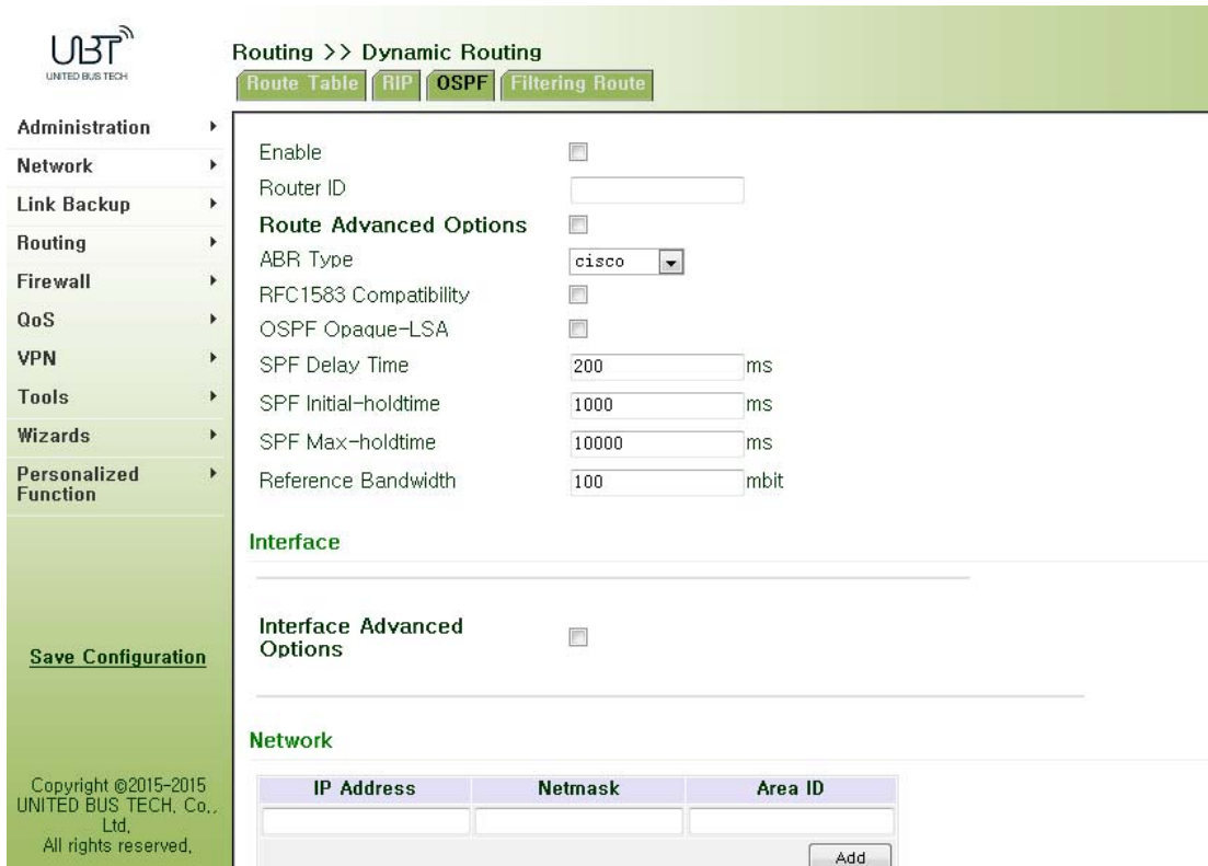
Figure 3-60 OSPF
