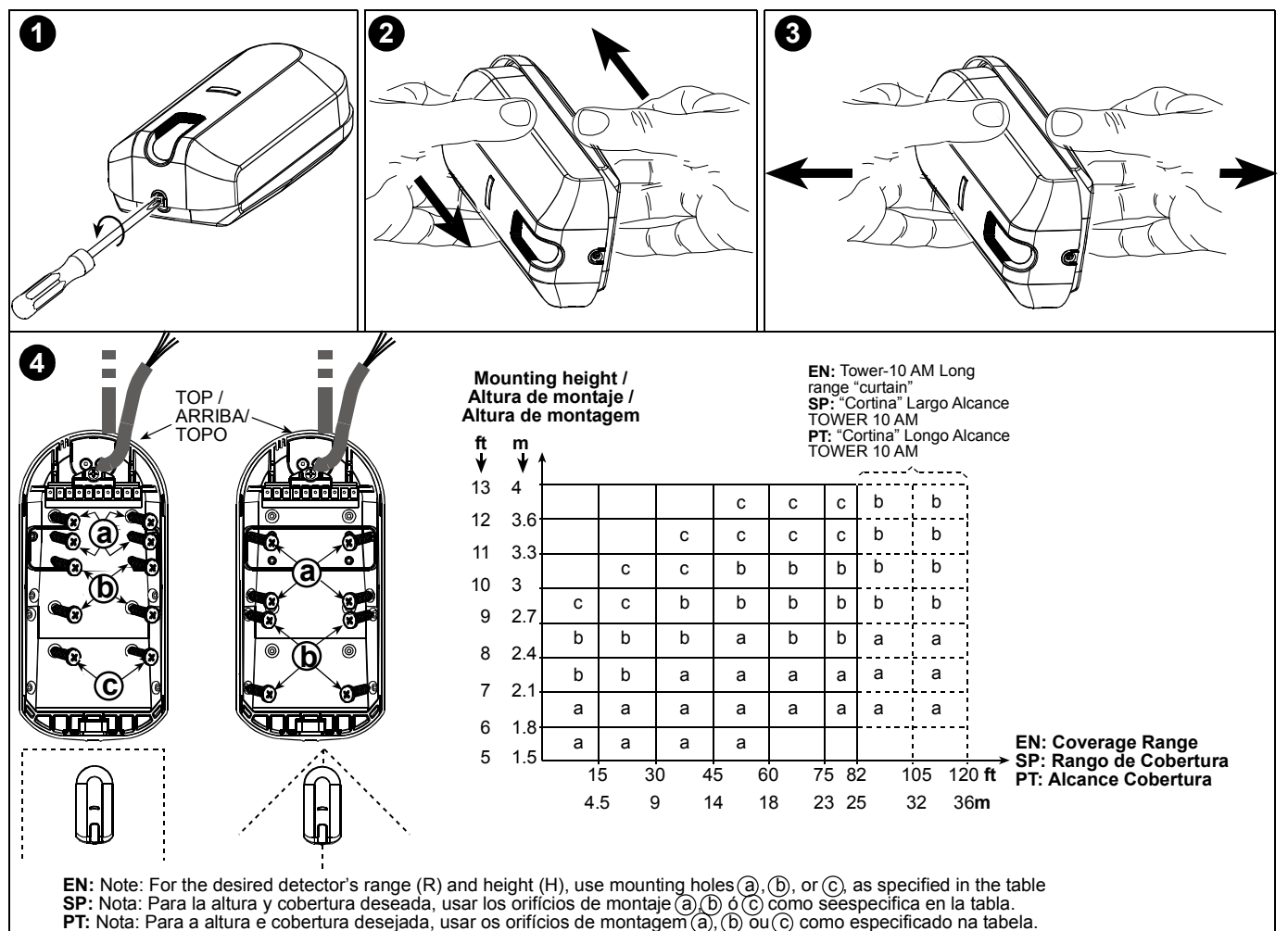
Fig. 4 - Mounting / Montaje / Montagem
