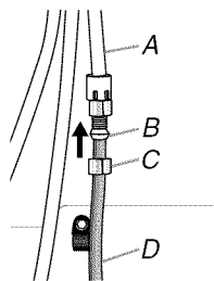
A. Tubería de agua de plástico C. Tuerca de compresión B. Manga D. Tubería de cobre
