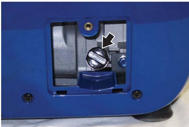
Figura 22 – Tapón de llenado/drenaje de aceite
