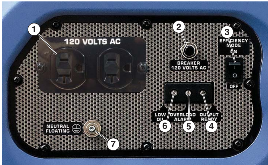
Figura 10 – Características del tablero de control
