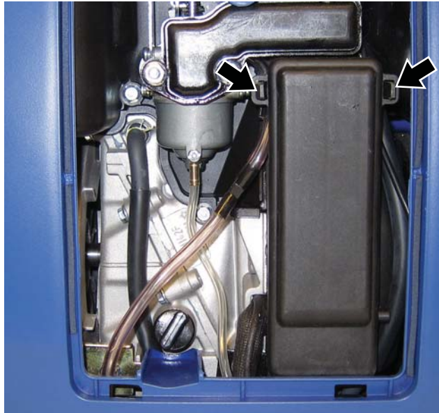
Figura 41 – Cubierta del filtro de aire
