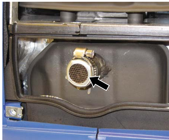
Figura 53 – Abrazadera del amortiguador de chispa
