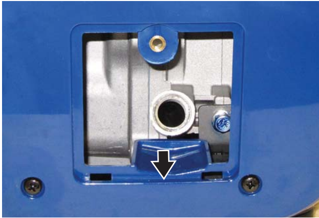
Figura 40 – Drene el aceite del motor
