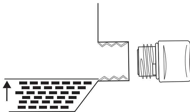
Figura 25 – Nivel correcto de aceite del motor
