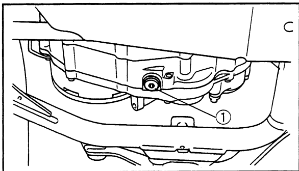
1. Drain plug (engine)
