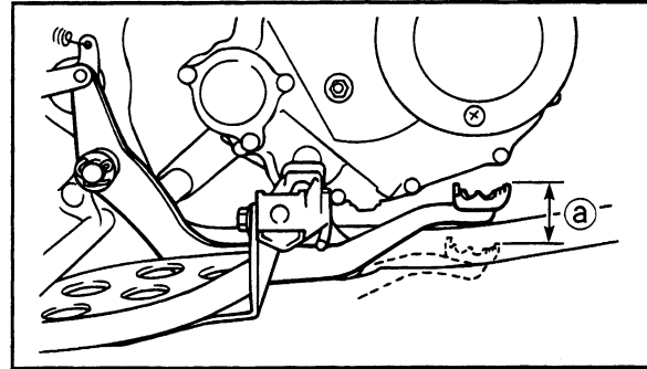
a. 20 ~ 30 mm (0.8 ~ 1.2 in)
