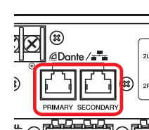
Conector [Dante] de la unidad MTX5-D/MRX7-D
