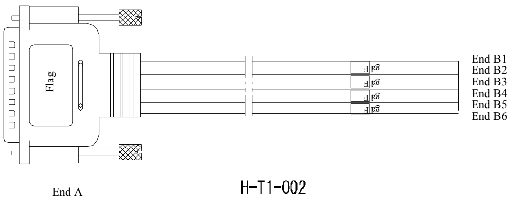
Fig. 7.4-1 100ΩT1 Cable Diagram
