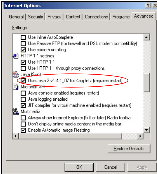
Figure 106 Java (Sun)
