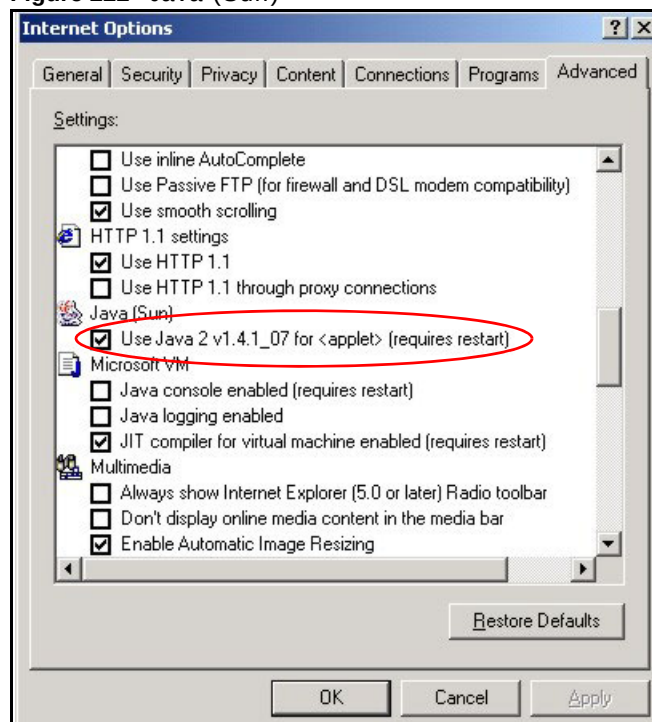
Figure 222 Java (Sun)
