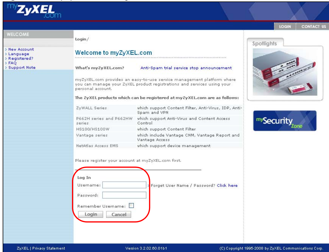
Figure 321 myZyXEL.com: Login
