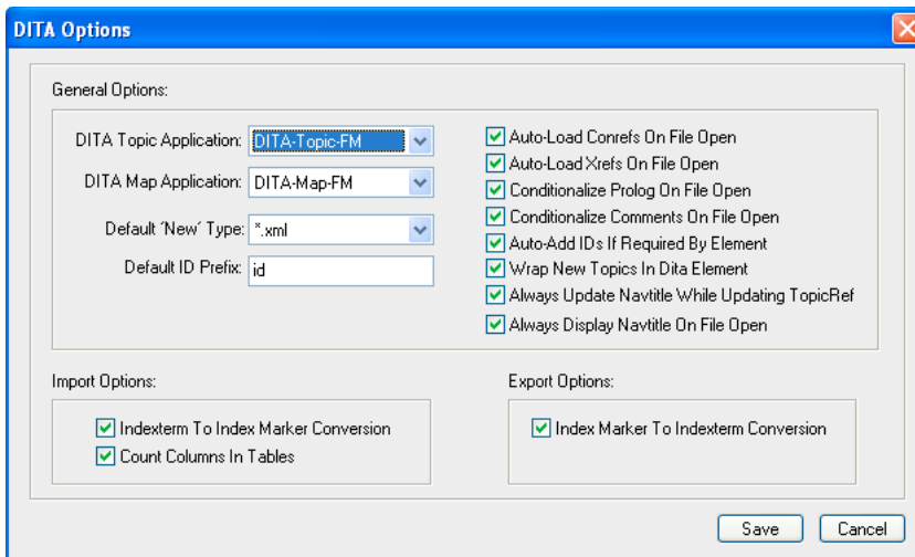
DITA options
