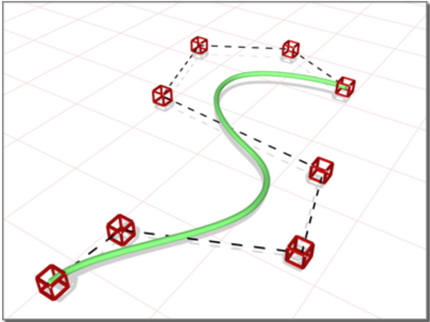
NURBS CV curve
