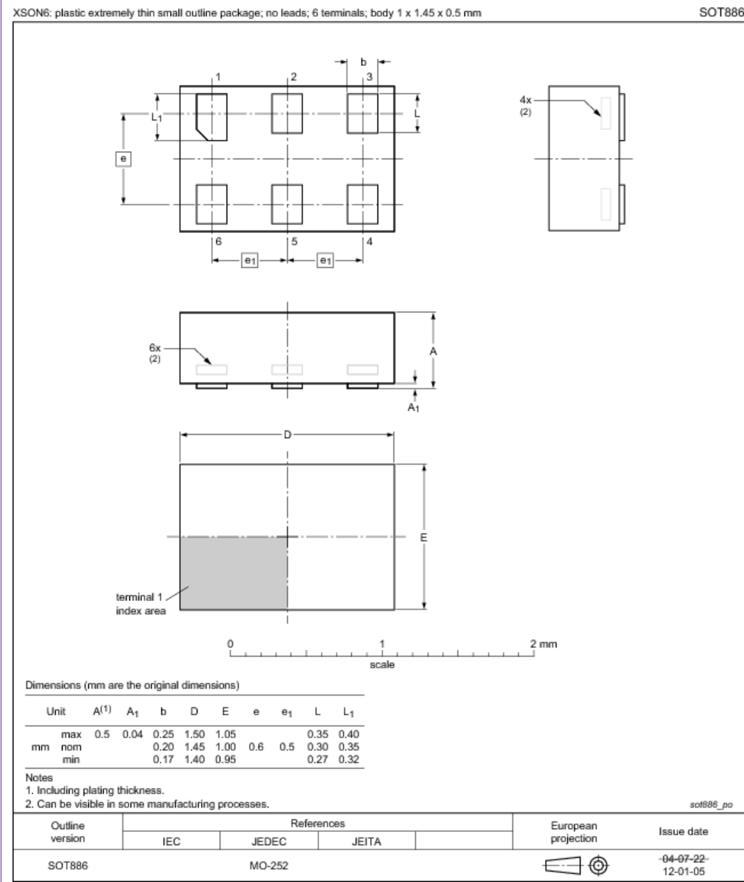
Fig 4. UCODE G2i SOT886
