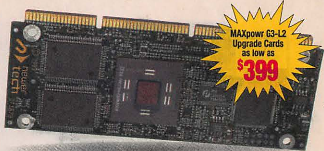
▲ MAXpower G3-L2
