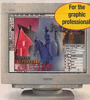
▲ Sony 500PS
