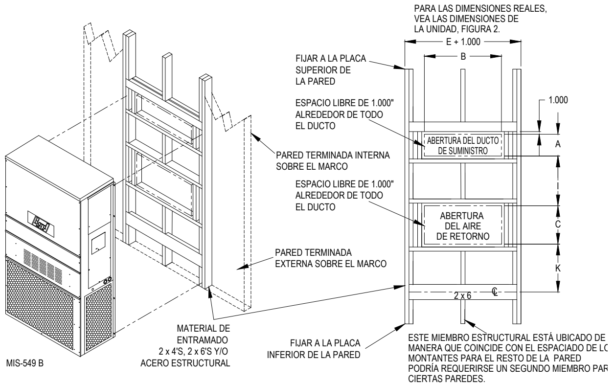
FIGURA 6 Instrucciones para montaje en pared
