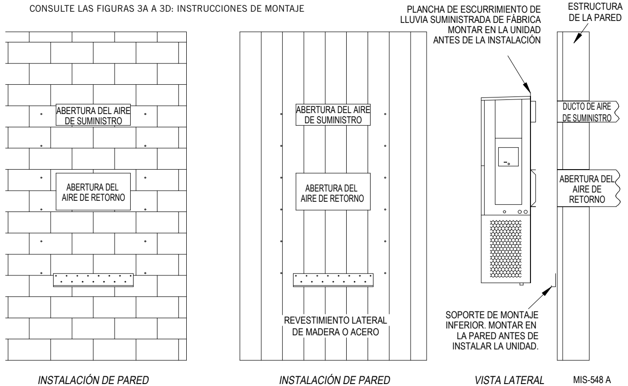
FIGURA 6 Instrucciones para montaje en pared
