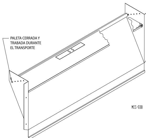
FIGURA 1 Regulador de aire exterior
