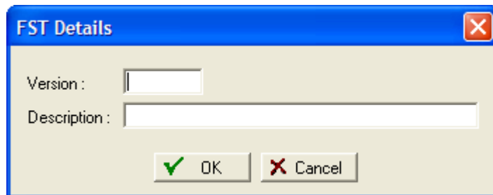
Figure 4-8. FST Details
