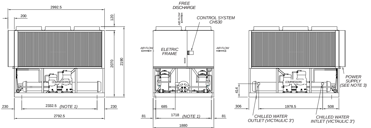
Fig. 17 - Unit Dimensions - CGAD 050
