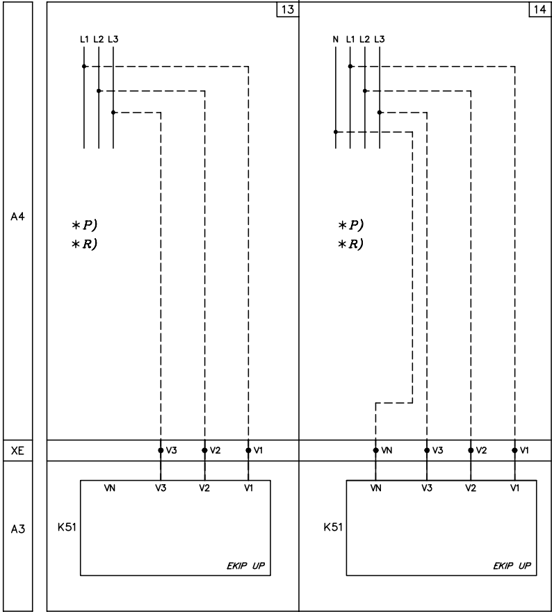
13) Ekip UP sin transformador de tensión externo y configuración 3P 14) Ekip UP sin transformador de tensión externo y configuración 4P
