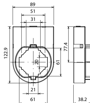
Sensor de corriente tipo B hasta 2500 A
