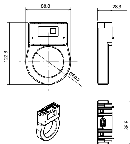
Sensor de corriente tipo B hasta 2500 A
