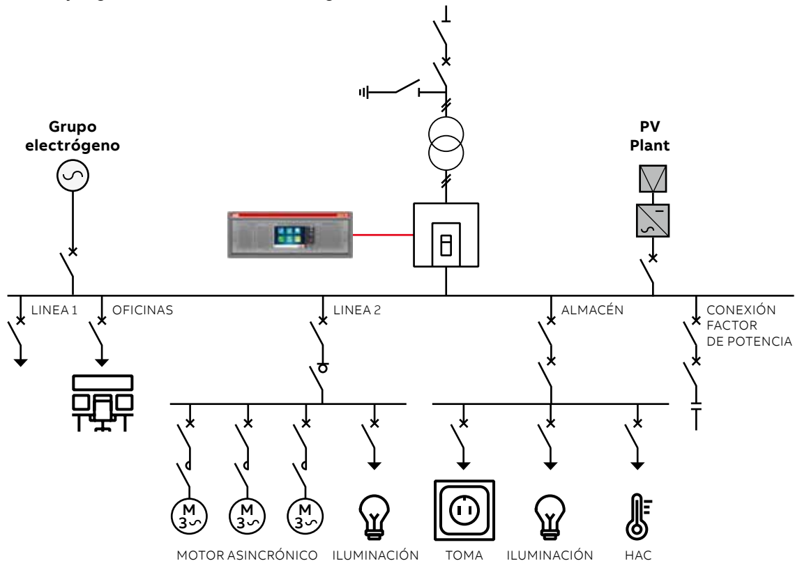
Aplicación típica de deslastre de las cargas
