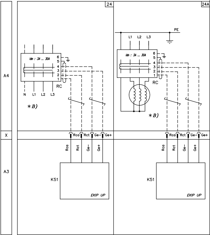
24) Entrada sensor protección de corriente residual RC (ANSI 64&50NTD) 24A) Entrada sensor de protección contra defecto a tierra diferencial RC (ANSI 87N)
