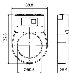
Sensor de corriente tipo B hasta 1600 A
