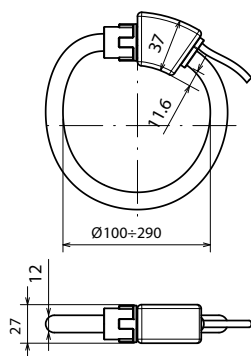
Sensor de corriente tipo C \varnothing 100-120-200 mm hasta 4000 A \varnothing 290 mm de 2000 A a 6300 A
