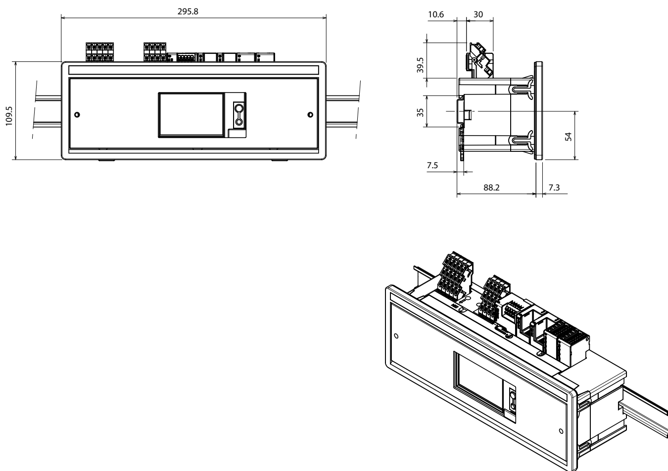
Unidad Ekip UP, montaje en perfil DIN, con módulos/terminales
