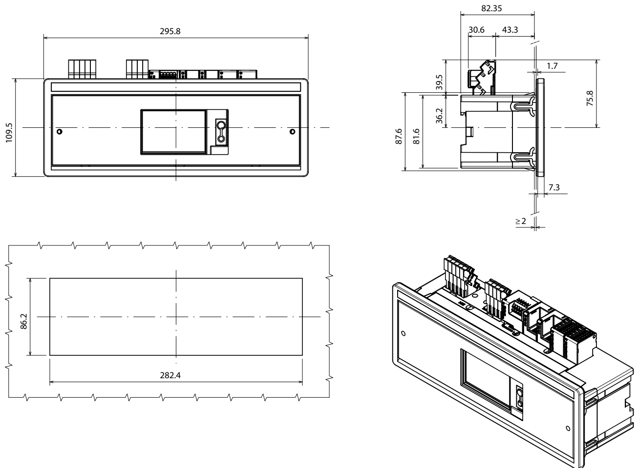
Unidad Ekip UP, montaje en la puerta, con módulos/terminales
