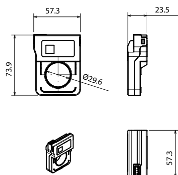
Sensor de corriente tipo B 100A-400A
