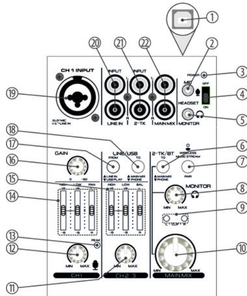
MicroMix 2 USB
