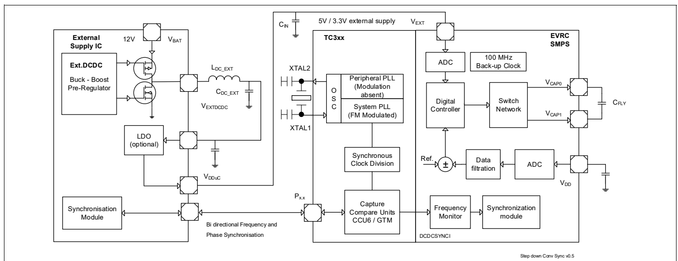
Figure 135 EVRC Synchronization Input
