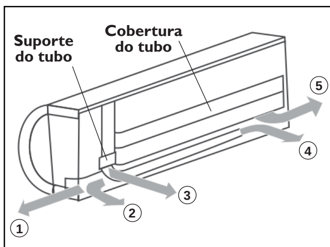
FIG. 9 - DIREÇÕES DAS TUBULAÇÕES
