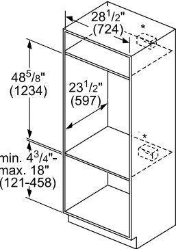
Cutout Dimensions
