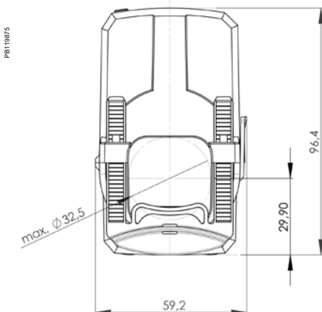
HG Dimensions
