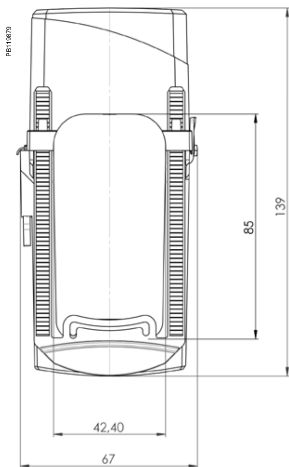
HM Dimensions
