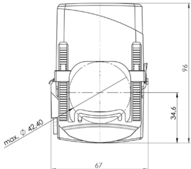
HJ Dimensions
