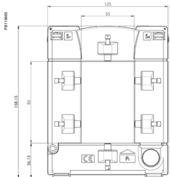
GD Dimensions
