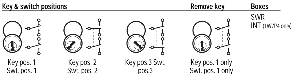
1W7R4—four switches
