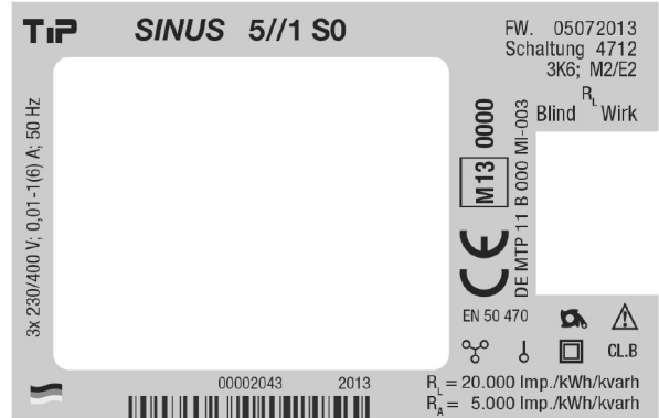
Exemple de plaque signalétique pour SINUS 5//1 S0
