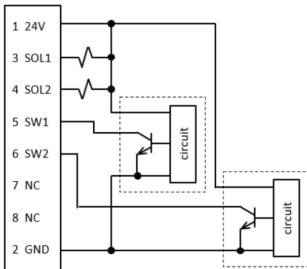
NPN output
