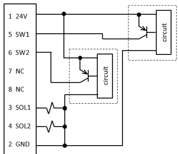
PNP output
