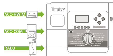
Componentes de comunicación de ACC para montaje de pared
