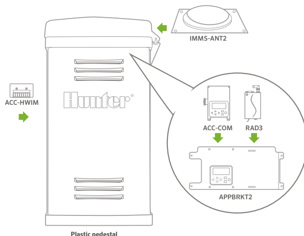
Componentes de comunicación de ACC para pedestal de plástico
