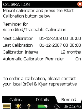
Fig. 5.6 Calibration reminder tab
