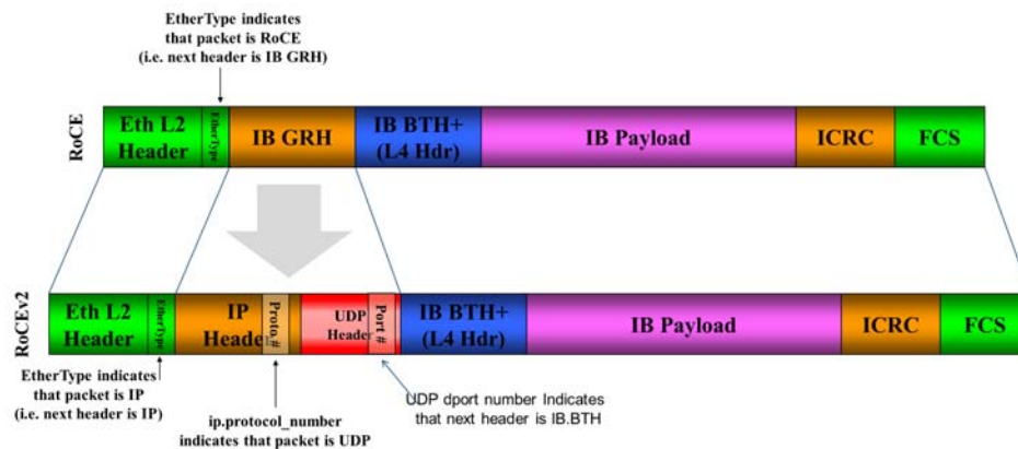
Figure 2: RoCE and RoCE Frame Format Differences
