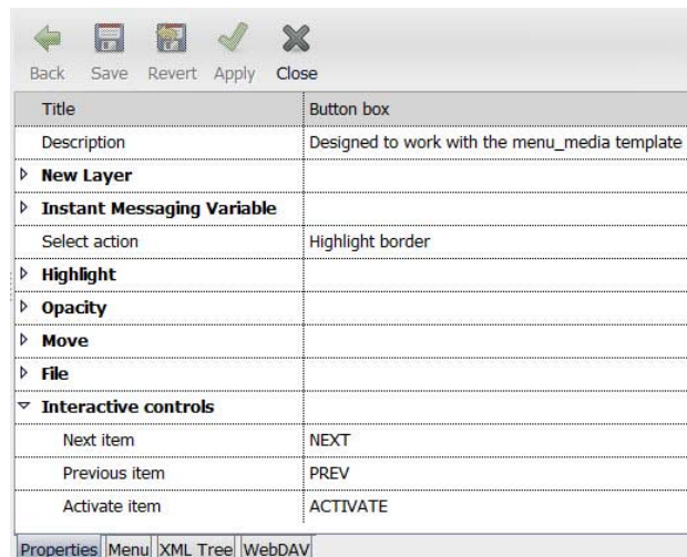
FIG. 76 Properties tab
