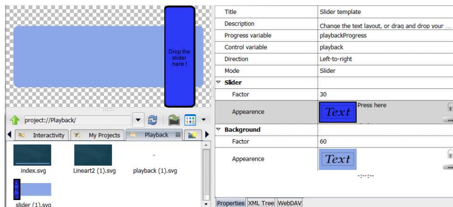
FIG. 93 Slider.svg properties
