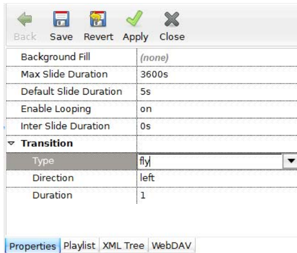
FIG. 17 Properties Tab
