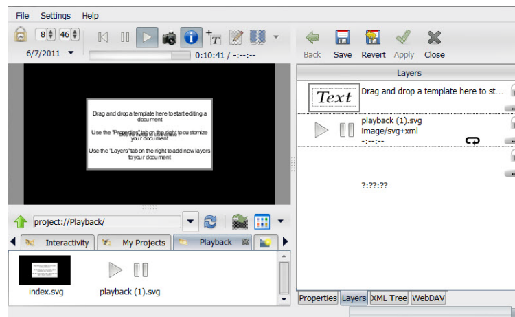
FIG. 87 Playback.svg
