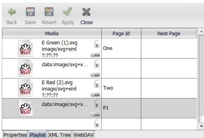
FIG. 68 Page ID
