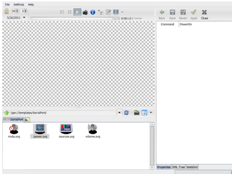
FIG. 114 Power.svg file
