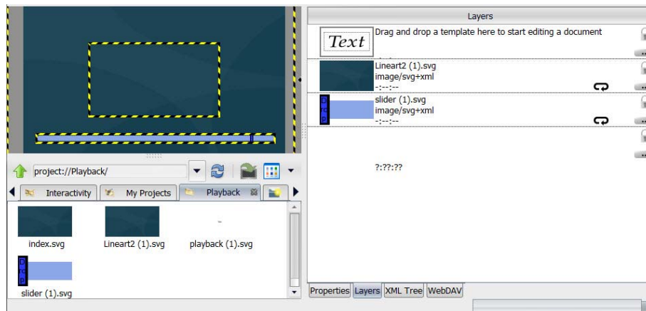
FIG. 92 Slider.svg placement
