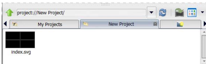
FIG. 54 Multiscreen index.svg
