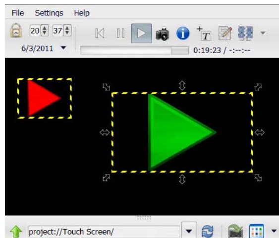
FIG. 70 Editing enabled
