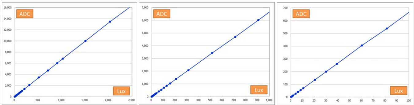
ALS ADC count vs. Lux @ASC_Normal mode with ASC_Gain=x1
