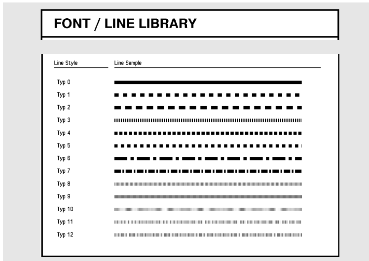
Fig. 28: Printer-internal line styles (Info-printout INFO AUSDRUCKEN > Font Status or Info > Status Ausdrücke > Font Status , section „Font /Line Library“).
