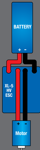
XL-5 HV Wiring Diagram
