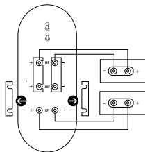
Bi-amp wiring
