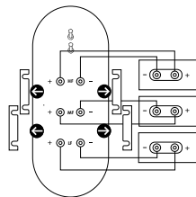
Tri-amp wiring
