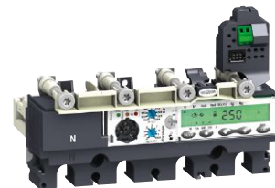
Micrologic-Auslöseeinheit für 4-polige Compact-Leistungsschalter
