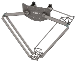
Delta 2 Greifermechanismus
