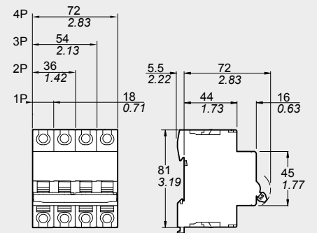
Abmessungen (mm / Zoll)
