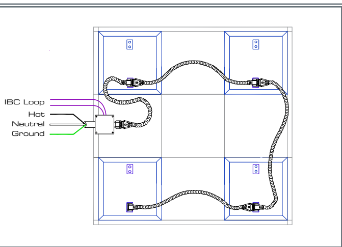
RELOC WIRING SYSTEM
