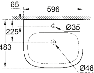
39 337 000 39 337 00H* Vasque à poser 60 cm
