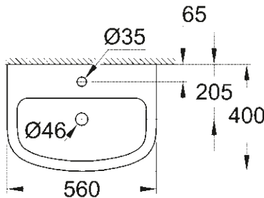
39 422 000 Lavabo à encastrer par le dessus 55 cm
