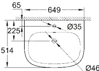
39 323 000 39 323 00H* Lavabo suspendu 65 cm
