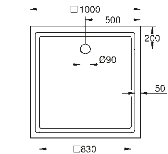
39 300 000* Bac de douche universel 100 cm x 100 cm
