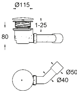
49 534 000* Clapet de vidage horizontal pour bacs de douche universels
