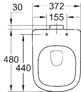
39 329 000 39 329 00H* WC posé au sol sans rebord
