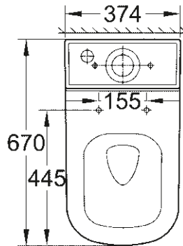
39 338 000 WC posé au sol pour combinaison monobloc Triple Vortex, sortie universelle
