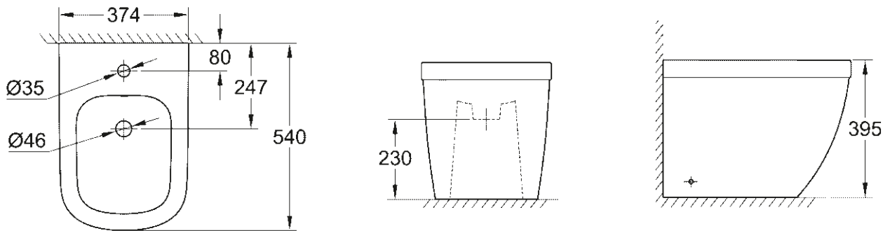
39 340 000 39 340 00H* Bidet posé au sol
