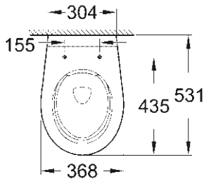
39 427 000 WC suspendu sans rebord
