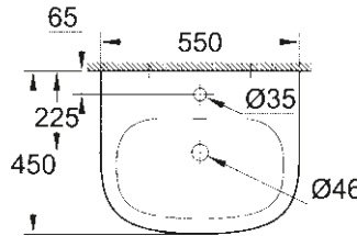
39 336 000 39 336 00H* Lavabo suspendu 55 cm
