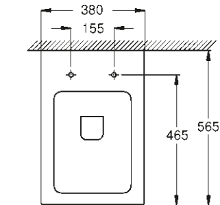
39 485 00H WC posé au sol contre paroi sans rebord
