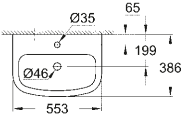
39 440 000 Lavabo suspendu 55 cm
