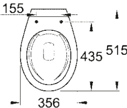
39 430 000 WC posé au sol sans rebord
