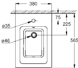
39 486 00H Bidet suspendu
