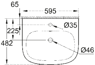
39 335 000 39 335 00H* Lavabo suspendu 60 cm
