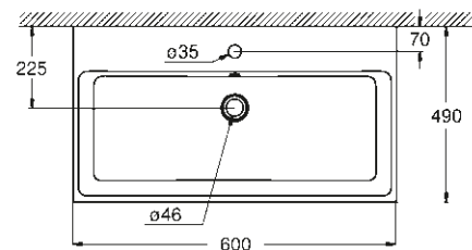
39 477 00H Vasque à poser 60 cm
