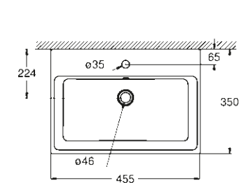
39 483 00H Lave-main 45 cm
