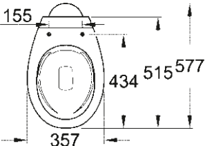
39 431 000 WC posé au sol sans rebord
