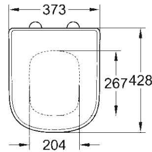
39 458 000 Siège et abattant avec frein de chute pour WC compact fonction déclinable
