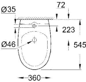
39 432 000 Bidet posé au sol
