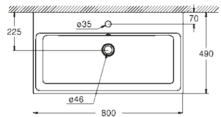
39 476 00H Vasque à poser 80 cm
