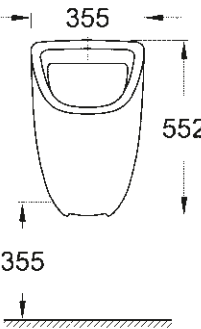
39 439 000 Urinoir avec entrée par le haut
