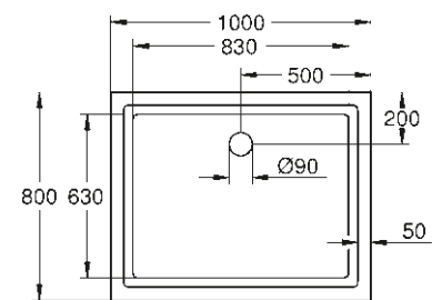
39 306 000* Bac de douche universel 80 cm x 100 cm
