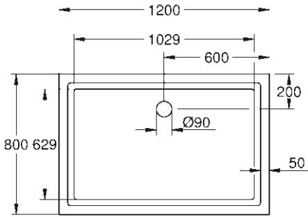
39 305 000* Bac de douche universel 80 cm x 120 cm
