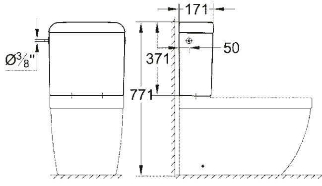
39 531 000 Réservoir de chasse avec entrée latérale et arrière, NF
