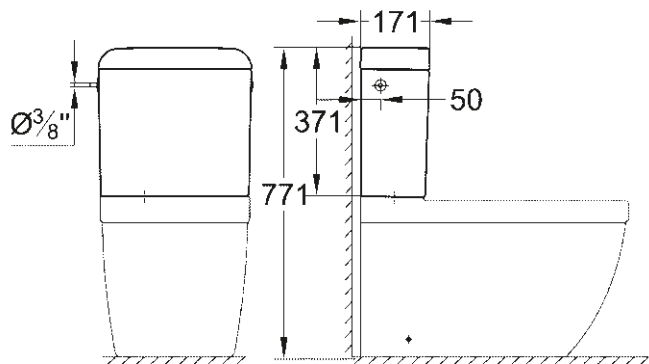
39 333 000 Réservoir de chasse avec entrée latérale et arrière
