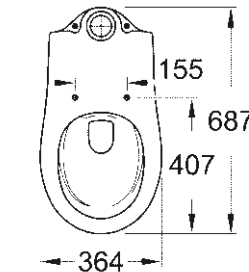
39 429 000 WC posé au sol pour combinaison monobloc sans rebord, sortie verticale
