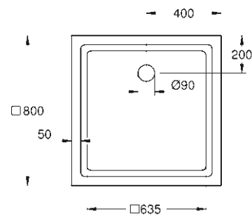
39 302 000* Bac de douche universel 80 cm x 80 cm
