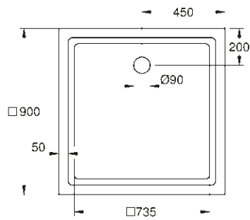
39 301 000* Bac de douche universel 90 cm x 90 cm
