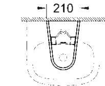
39 325 000 Demi-colonne pour lave-main 45 cm
