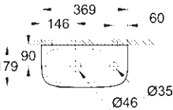
39 327 000 39 327 00H* Mini lave-main 37 cm
