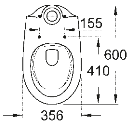
39 349 000 WC posé au sol pour combinaison monobloc sans rebord, sortie horizontale 39 428 000 rebord cloisonné
