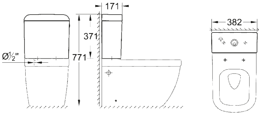
39 332 000 Réservoir de chasse avec entrée par le bas
