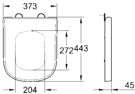
39 330 000 Siège et abattant avec frein de chute fonction déclinable
