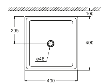
39 482 00H Vasque 40 cm
