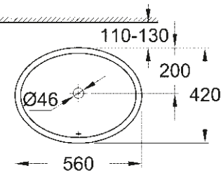
39 423 000 Vasque à encastrer par le dessus 55 cm
