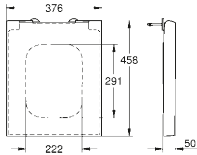
39 488 000 Siège et abattant avec frein de chute fonction déclinable
