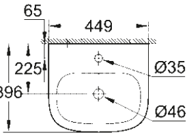
39 324 000 39 324 00H* Lave-main 45 cm
