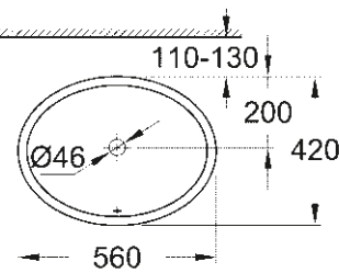
39 423 000 Vasque à encastrer par le dessus 55 cm
