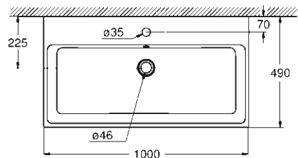
39 475 00H Vasque à poser 100 cm
