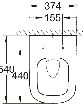
39 339 000 39 339 00H* WC posé au sol contre paroi sans rebord
