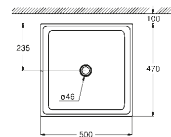
39 481 00H Vasque 50 cm
