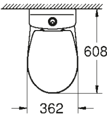
39 347 000 WC pour combinaison monobloc : WC, rebord cloisonné, sortie horizontale (39 428 000) Réservoir de chasse avec entrée latérale (39 437 000) Siège et abattant avec frein de chute (39 493 000) 39 495 000 Réservoir de chasse avec entrée latérale, NF (39 494 000) Siège et abattant (39 492 000)
