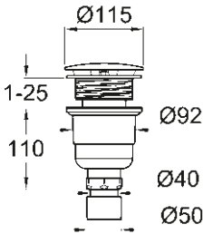
49 533 000* Clapet de vidage vertical pour bacs de douche universels
