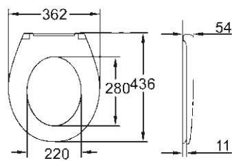
39 493 000 Siège et abattant avec frein de chute fonction déclinable 39 492 000 Sans frein de chute fonction déclinable
