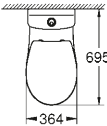
39 346 000 WC pour combinaison monobloc : WC, sans rebord, sortie verticale (39 429 000) Réservoir de chasse avec entrée latérale (39 437 000) Siège et abattant avec frein de chute (39 493 000) 39 496 000 Réservoir de chasse avec entrée latérale, NF (39 494 000)
