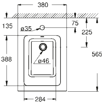
39 487 00H Bidet posé au sol
