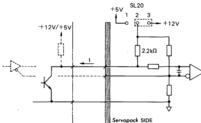
Fig. 6.4 Input Circuit (2)
