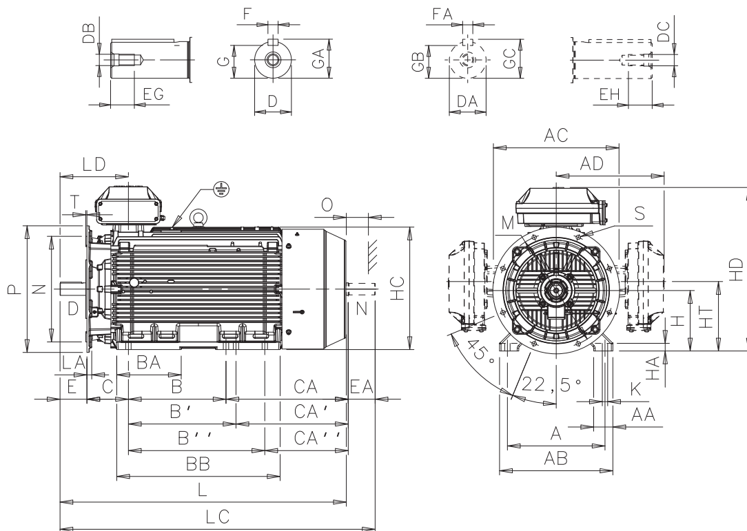
Mounting options IM B35 (IM 2001), IM V15 (IM 2011) and IM V36 (IM 2031).
