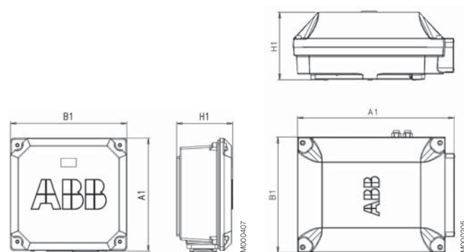
Fig. 1 Motor sizes 160 – 250
