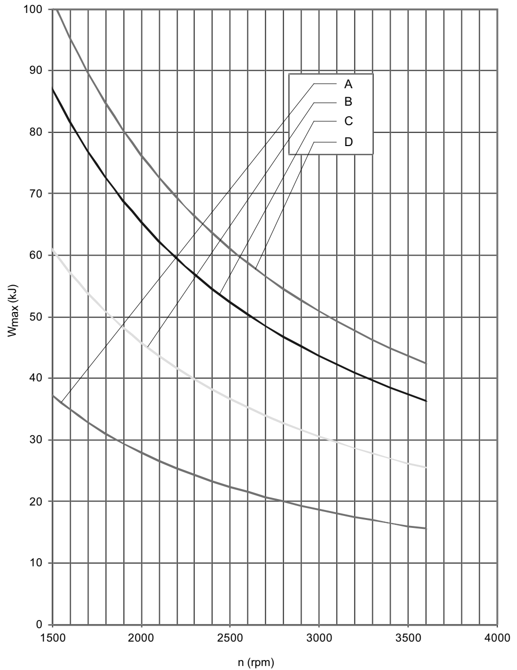
Diagram W_{\max} BE30:
