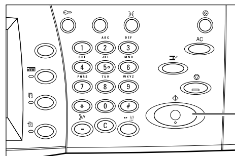
Botón <Comenzar>
