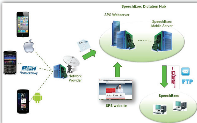
Diagrama del centro de dictados de Philips SpeechExec
