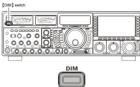
【DIM】 switch
