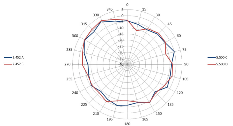
5.500 GHz
