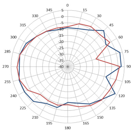
2.452 GHz
