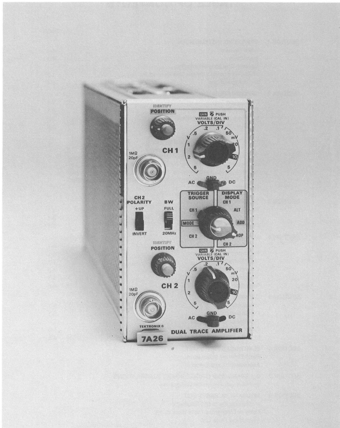
Fig. 1-1. 7A26 Dual Trace Amplifier.
