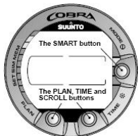
Figura 3.2. Pulsadores del ordenador de buceo.
