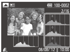
Histograma RGB
